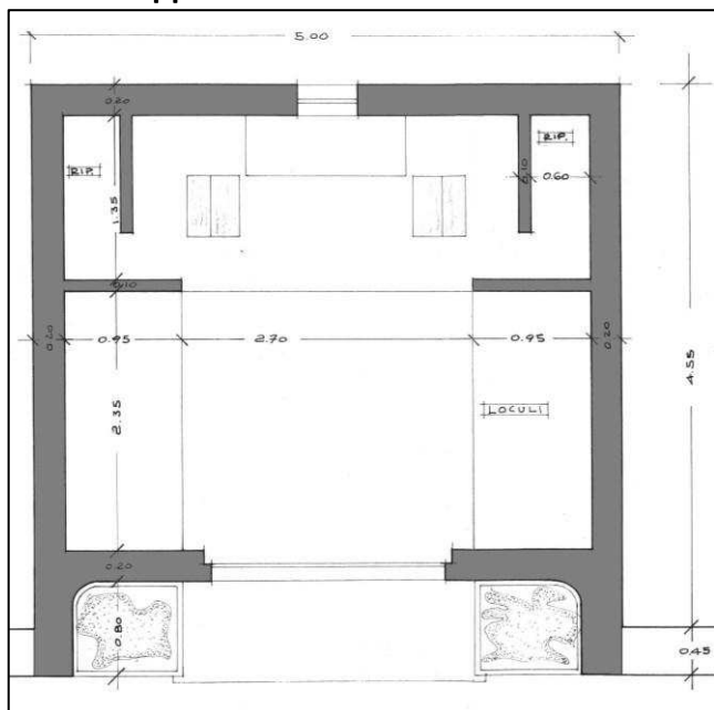
Pianta Cappella
